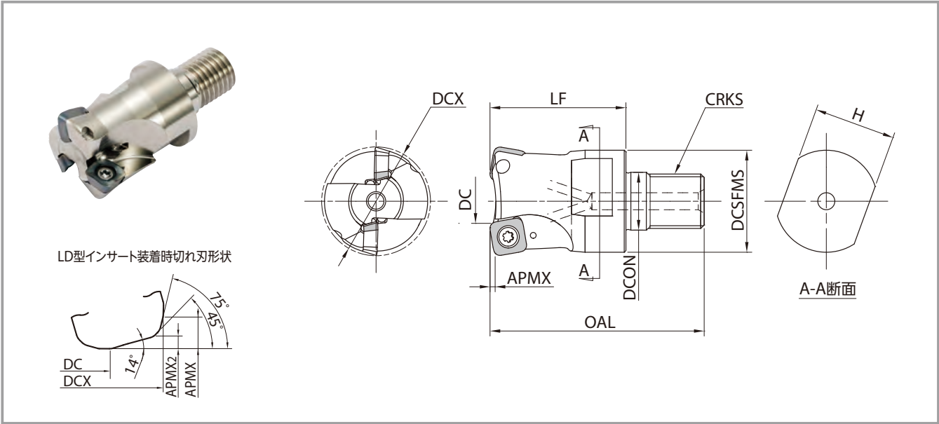
ホルダ寸法
