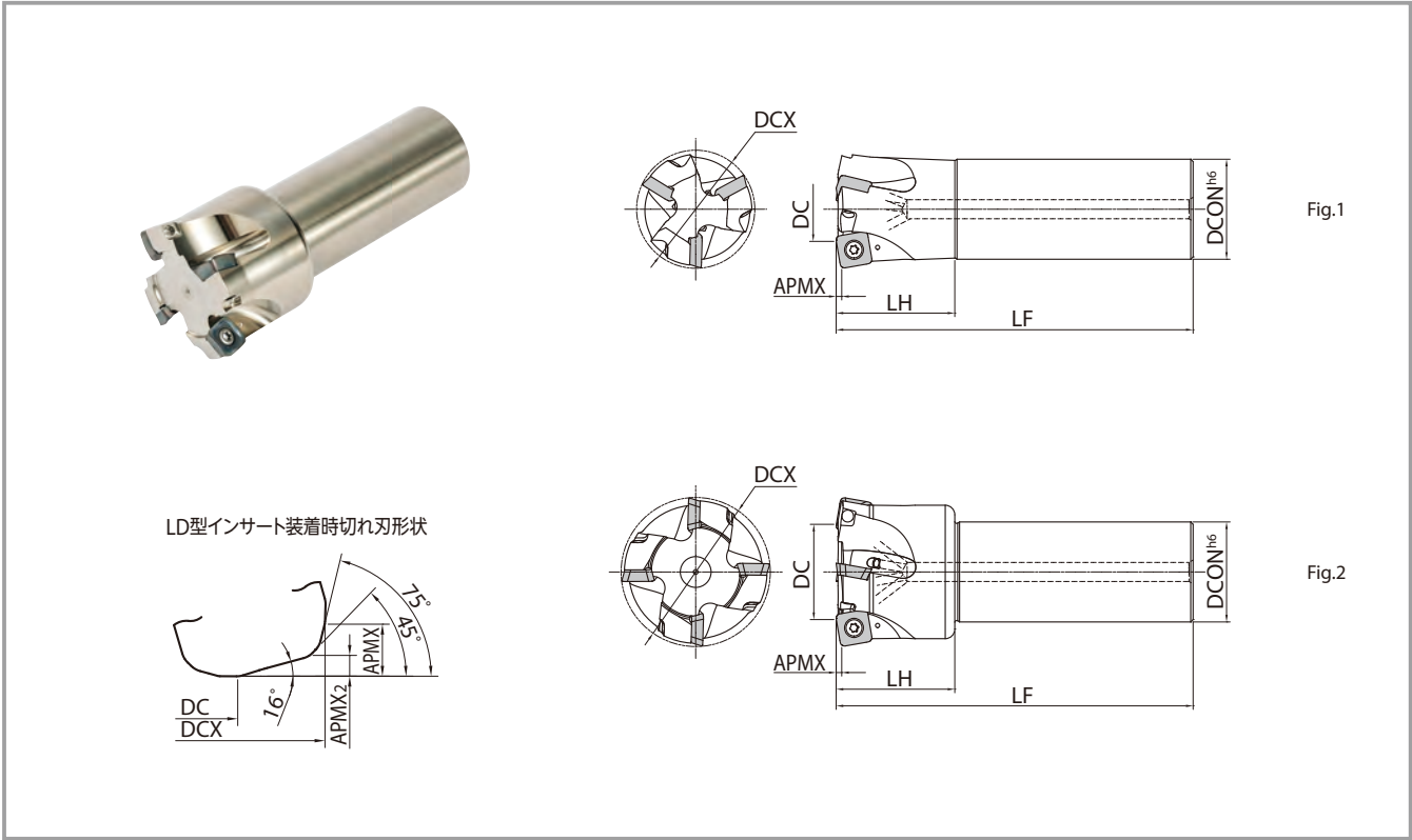
ホルダ寸法 (SOMT14タイプ)
