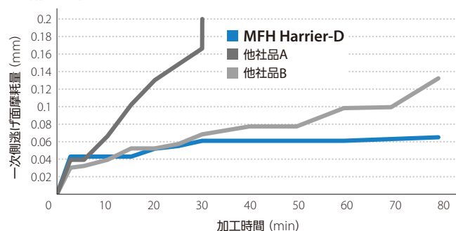
耐摩耗性比較 (当社比較)
