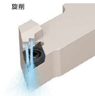
スクリューオン-JCTM
